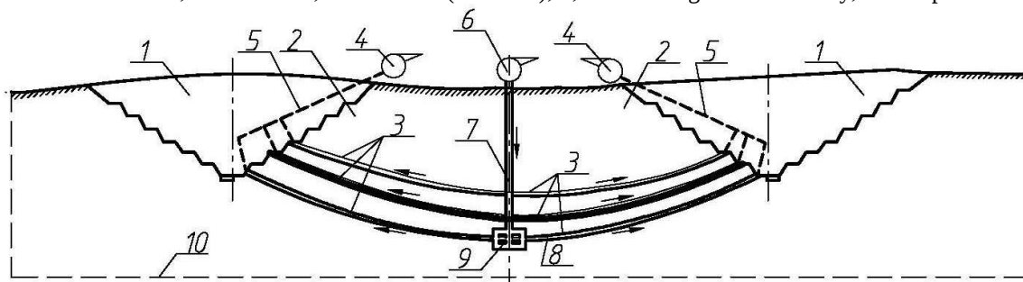
Рис. 6. Вентиляция подземных горных выработок при комбинированном способе разработки синклинальных угольных месторождений:
